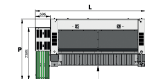
Empileur compact (roll-off)
